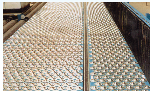
Zařízení skladu s hutními výrobky
