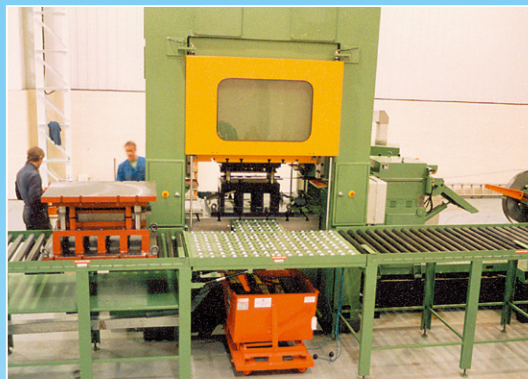
Kuličkový stůl před lisem pro rychlou výměnu tvářecích nástrojů
