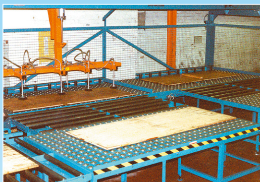
Nábytkářská výrobní linka
